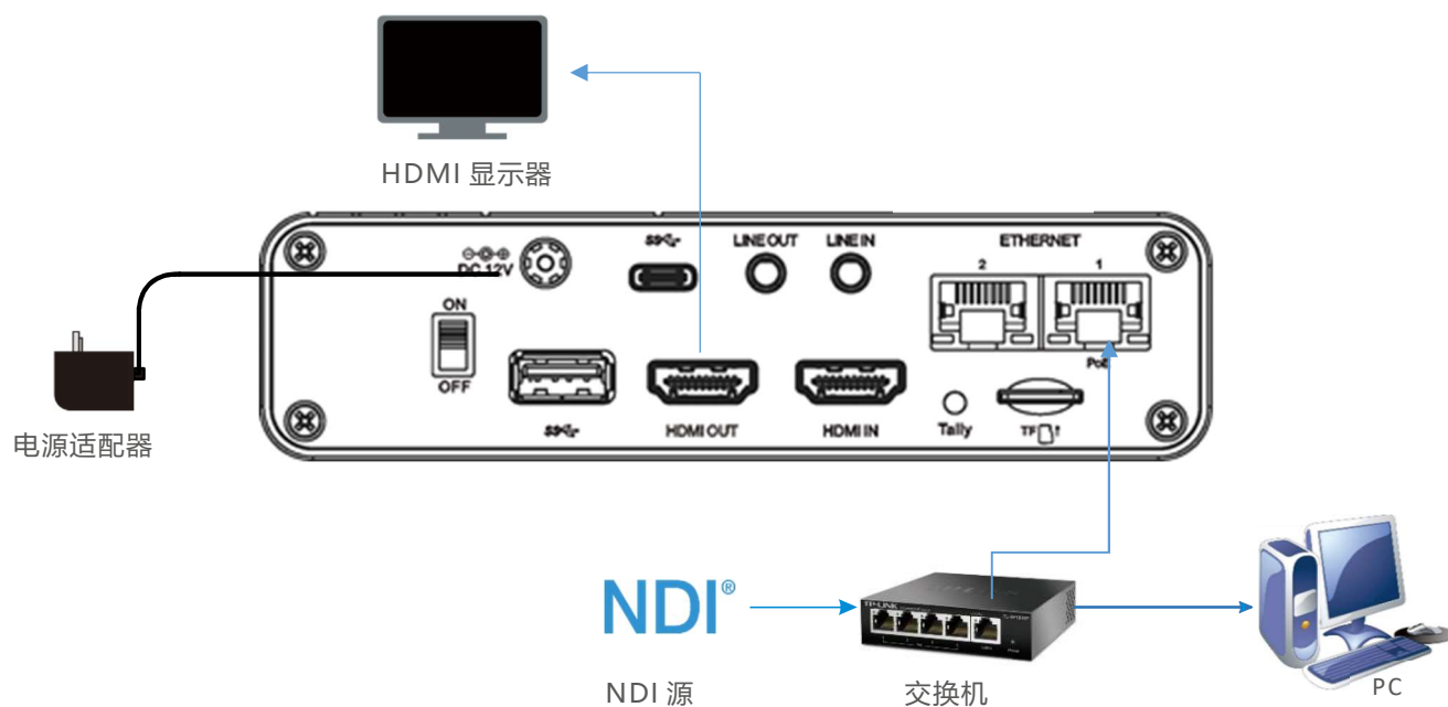
解码模式应用系统连接图
